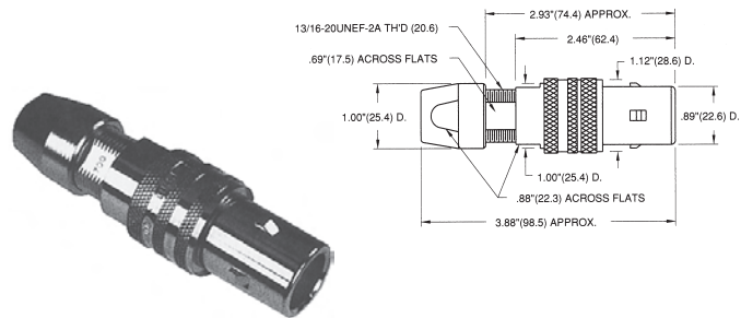
PLUG 7705-2 7705-3
