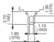
Solder lug
