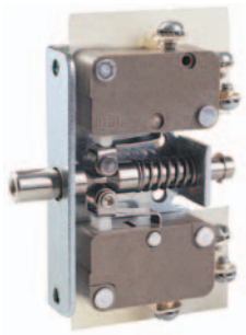
Door Interlock
