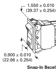
Snap-In Bezel
