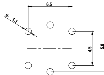
P.C.B LAND DIMENSION
