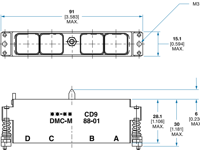
DMC-M 88-01: 4 Modules
