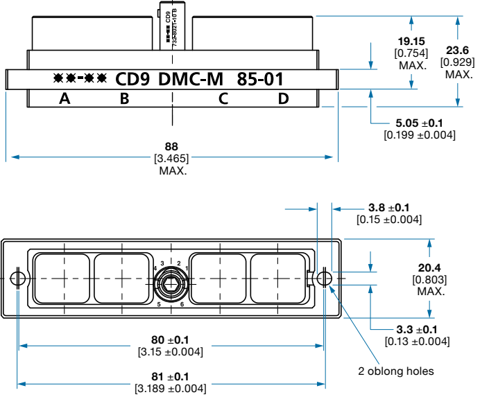
DMC-M 85-01: 4 Modules
