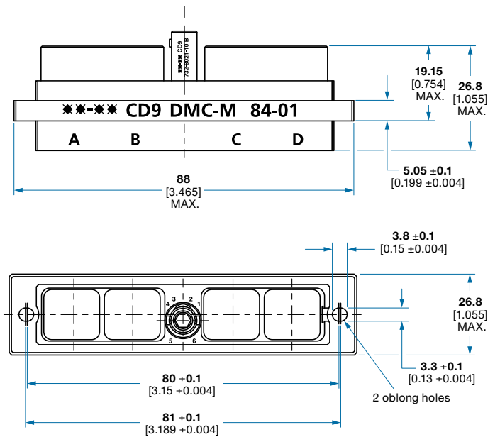
DMC-M 84-01: 4 Modules
