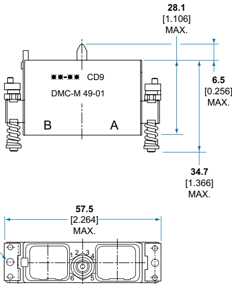
DMC-M 49-01: 2 Modules
