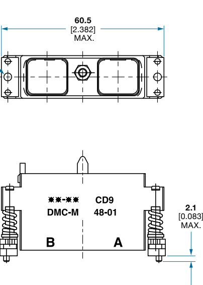
DMC-M 48-01: 2 Modules
