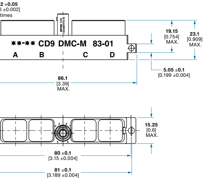
DMC-M 83-01: 4 Modules
