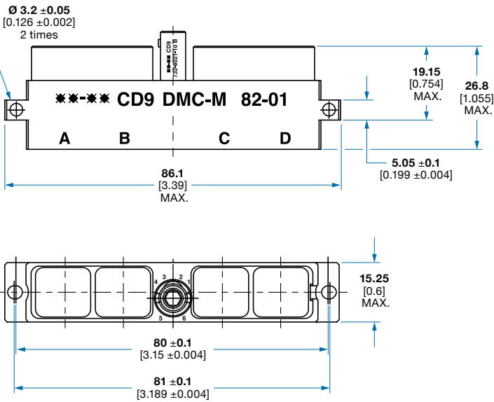
DMC-M 82-01: 4 Modules
