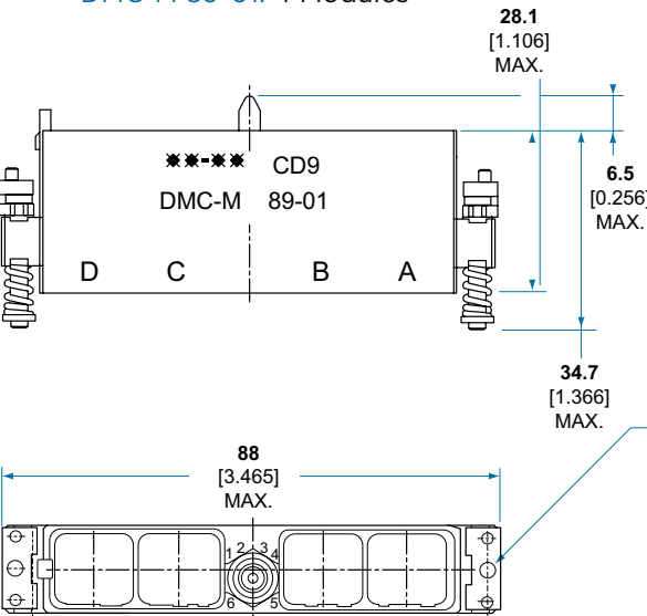
DMC-M 89-01: 4 Modules
