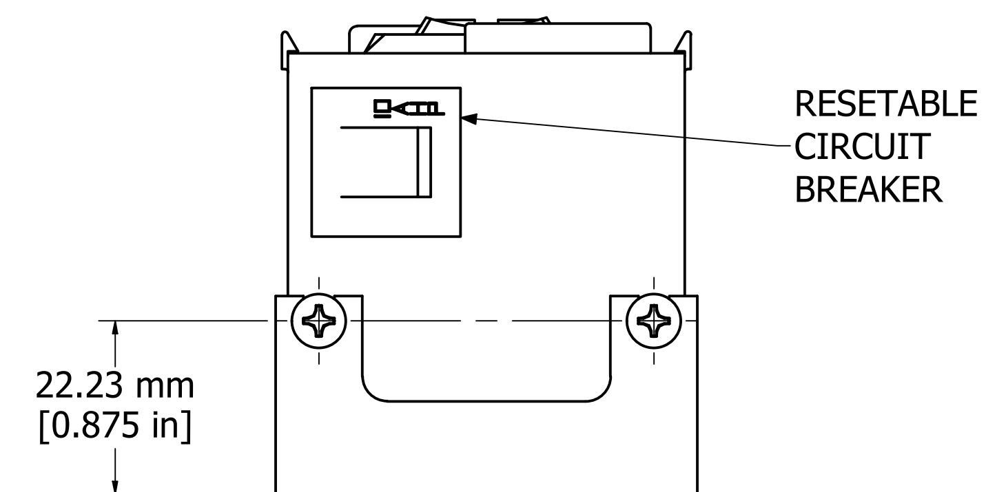
VIEW A-A
