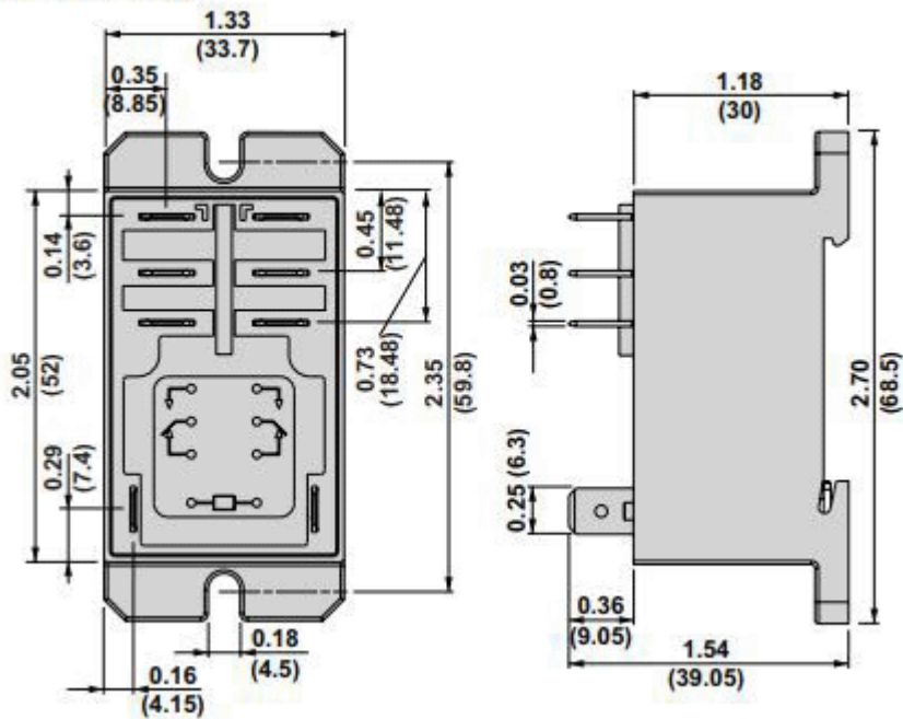
DPDT (2 CO):
