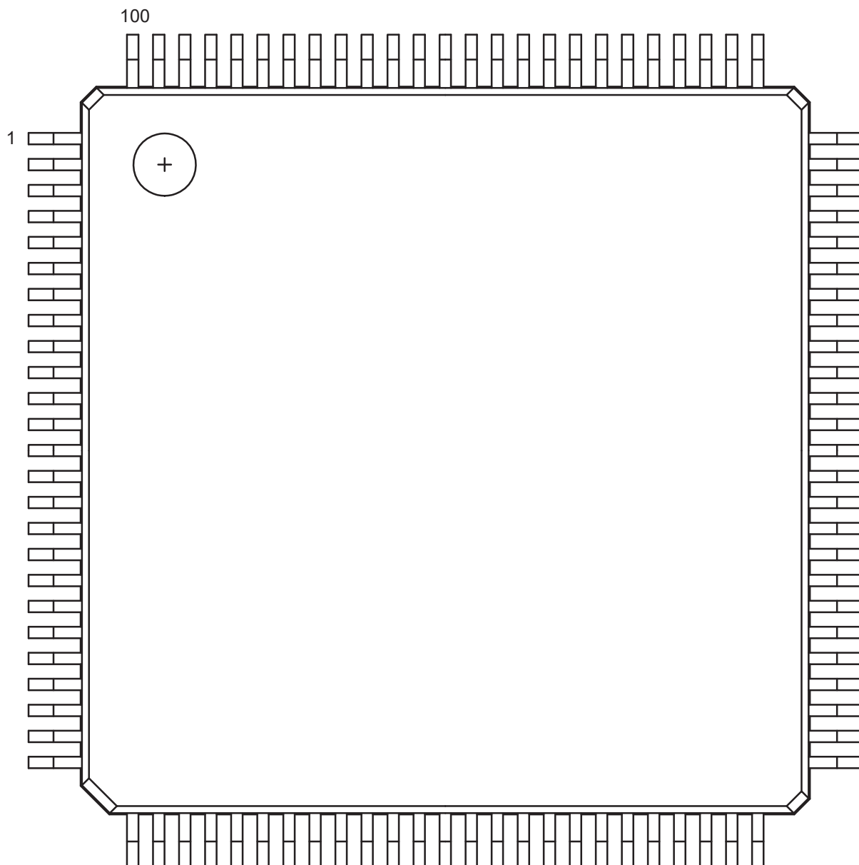
FIGURE 4-4 • VQ100—TOPVIEW
