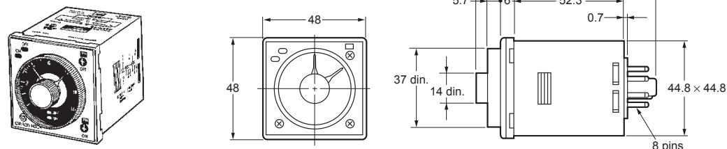
H3CR-F8 H3CR-F8N
