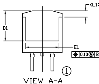
VIEW A-A
