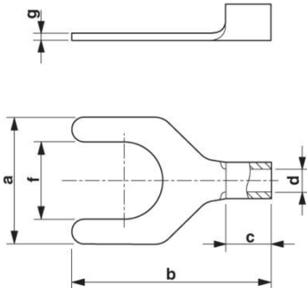
Maßzeichnung
