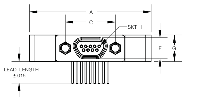
RECEPTACLE
