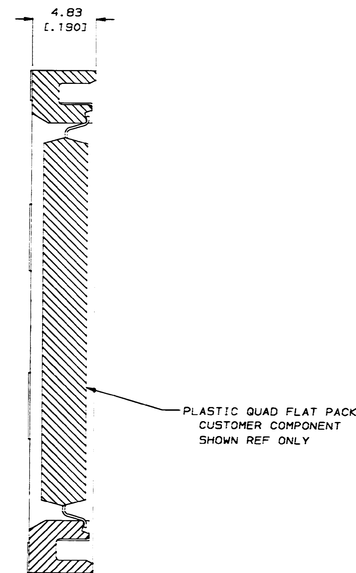
SECTION A-A
