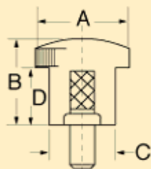
Projecting Stud
