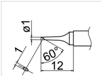
T12-C1 Shape-1C
