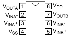
MCP662 SOIC
