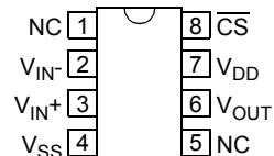
MCP663 SOIC
