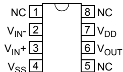
MCP661 SOIC
