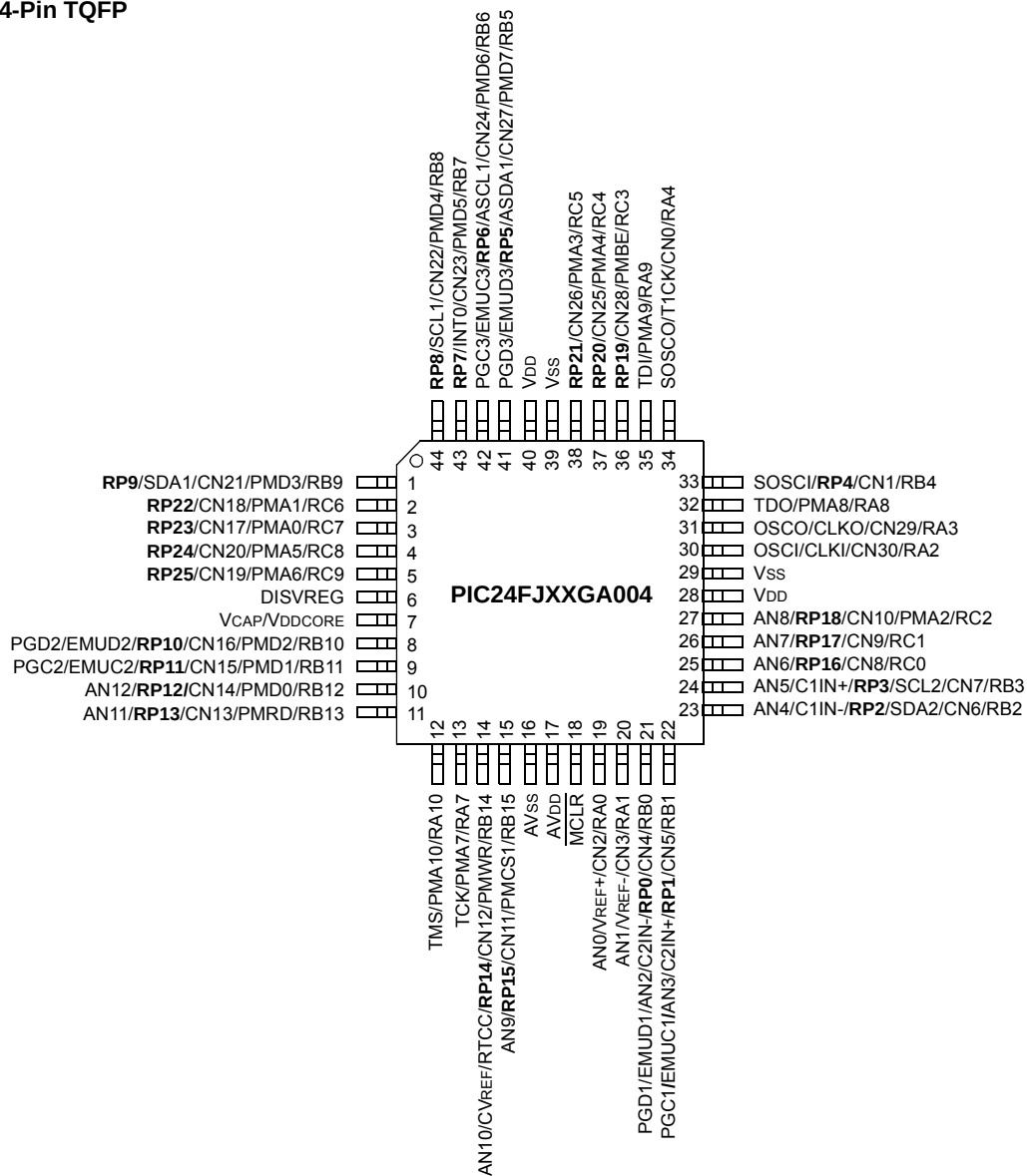
44-Pin TQFP
