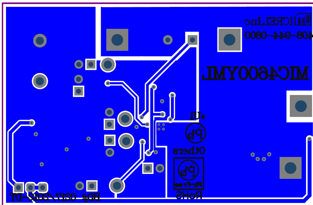
Bottom Layer
