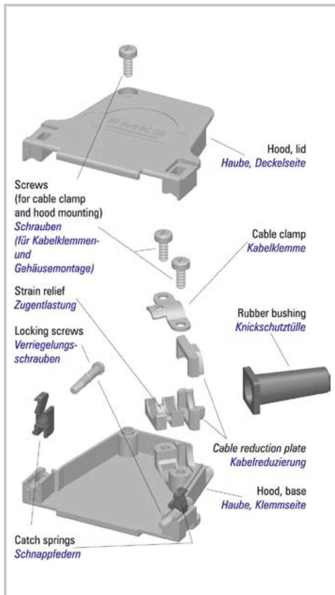
Metallhauben der Serie FMK in den Gehäusegrößen 1 - 5.
