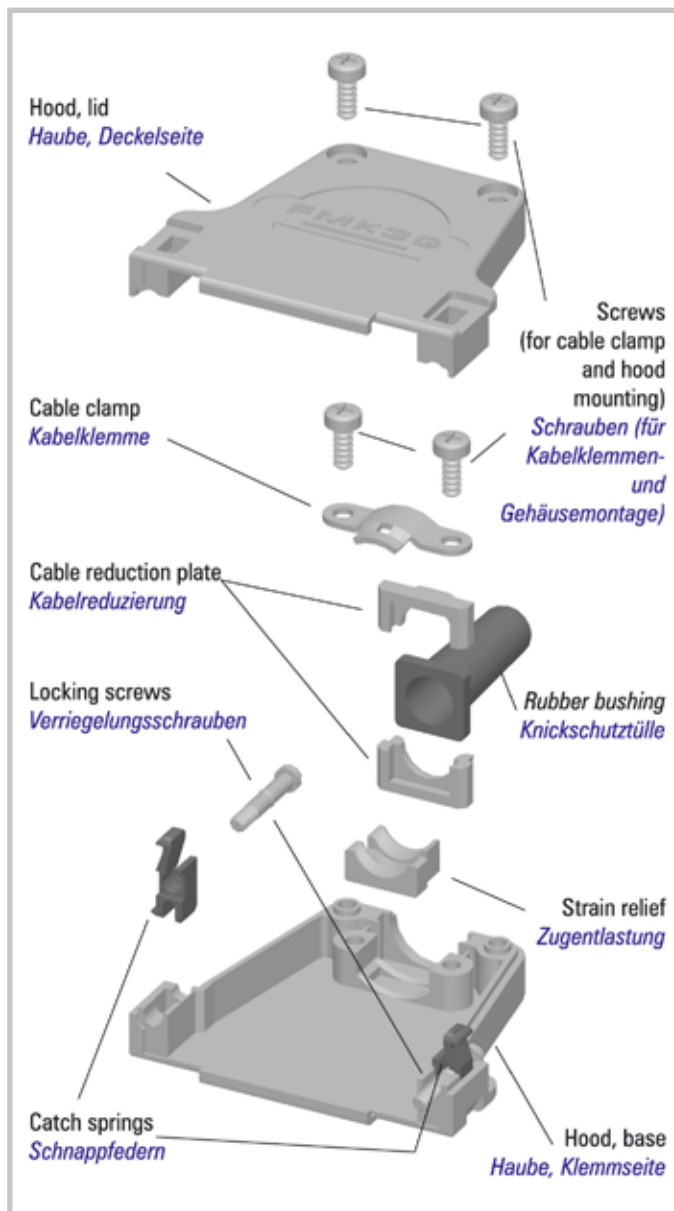
Metallhauben der Serie FMK...G in den Gehäusegrößen 1 - 5.
