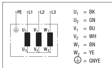
Star (3~ 400 VAC)
