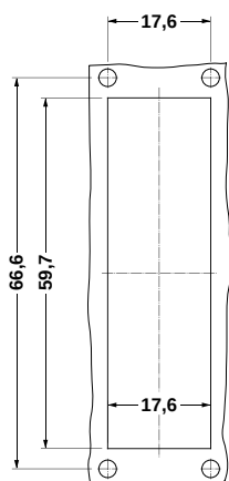
Panel cutout: VS-25-A
