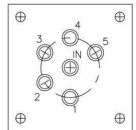
SP5T
