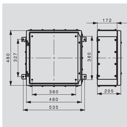
480 × 480 × 205 (18.90 × 18.90 × 8.07)
