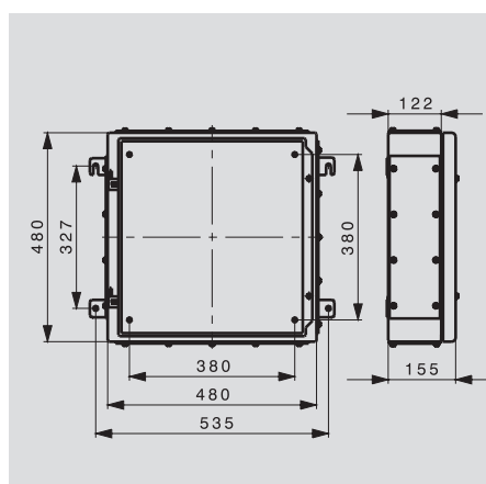
480 × 480 × 160 (18.90 × 18.90 × 6.30)
