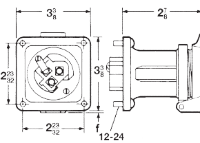
AR Receptacle – Spring Door
